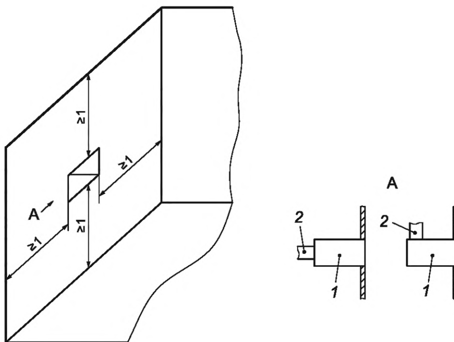
Рисунок 6 — Установка воздухораспределительного оборудования на ограждающей поверхности или напротив нее без воздуховода (см. ГОСТ 32549, [4] или [7])
