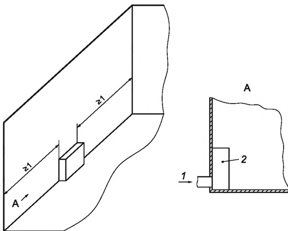
1 — бесшумная подача воздуха; 2 — испытуемое устройство
