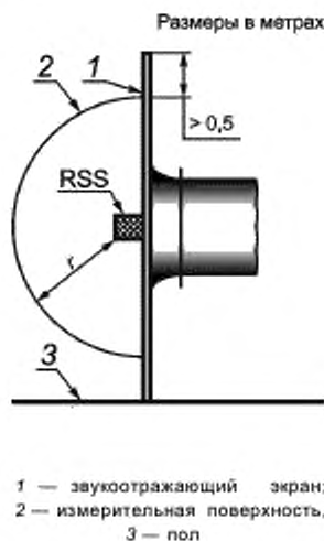
Рисунок А.1 — Определение показателя акустических условий K_2
