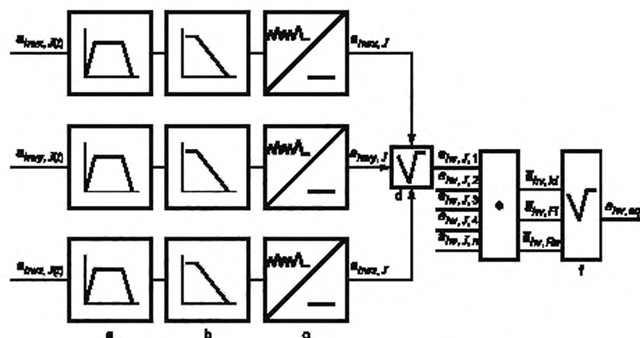
а — полосовой фильтр; б — весовой фильтр; в — измерение среднеквадратичного значения; д — вычисление полной вибрации; е — усреднение по всем измерениям для данного режима работы; ф — вычисление эквивалентной полной вибрации (см. А.4.2 и В.4.2)
