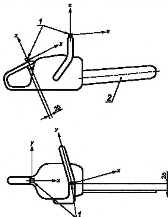
1 — акселерометры, 2 — осевая линия направляющей шины
