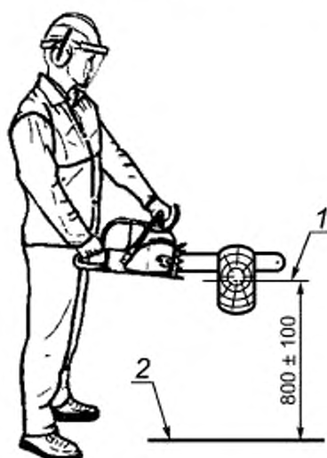
1 — ось бруса; 2 — уровень пола
