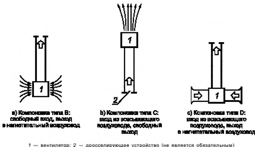
Рисунок С.1 — Компонировки вентилятора с воздуховодами
