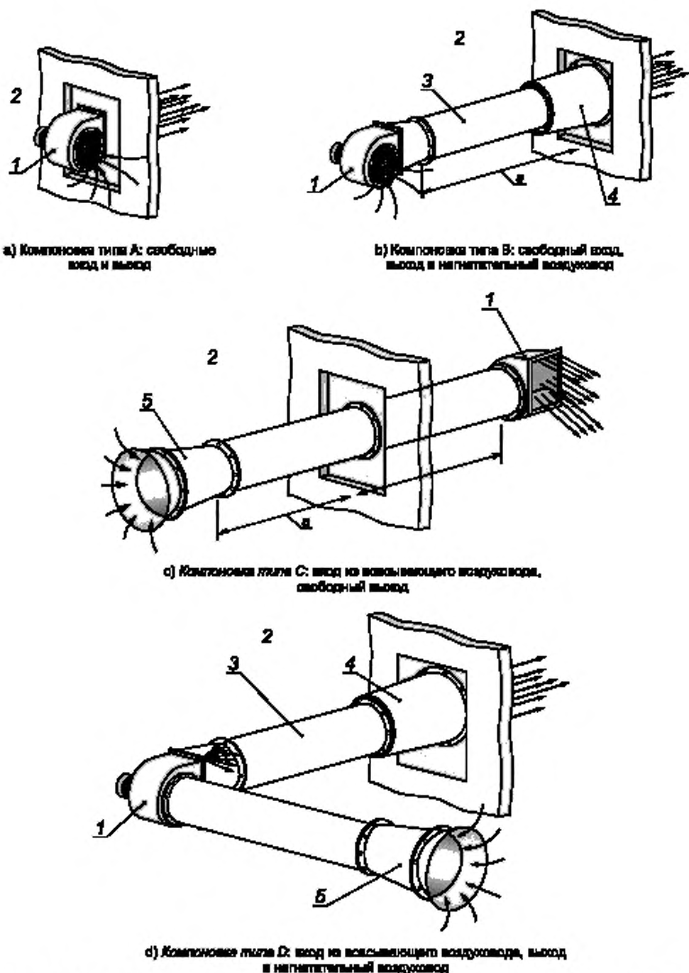
Рисунок 1 — Испытательная установка для измерений шума на входе вентилятора (показан радиальный вентилятор)
