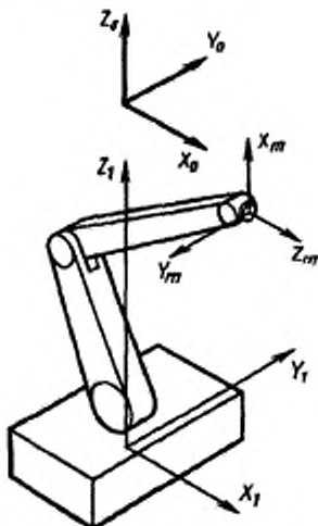
Рисунок 3 — Системы координат
