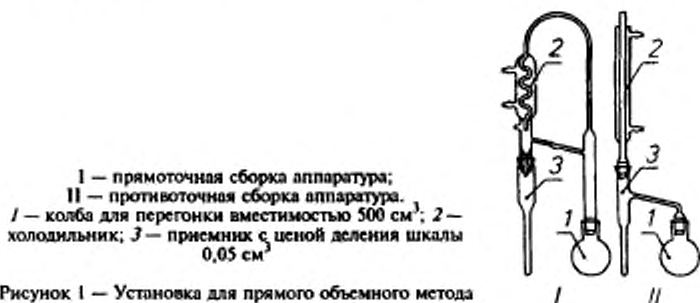
Рисунок 1 — Установка для прямого объемного метода определения влаги
