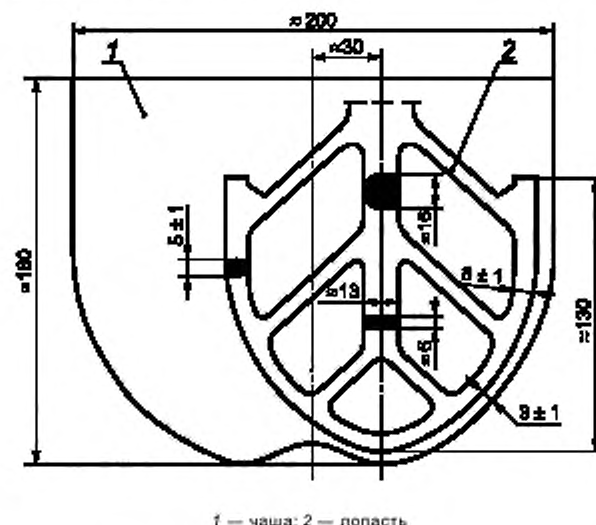
Рисунок 1 — Смеситель для приготовления растворов и мелкозернистых бетонных смесей
