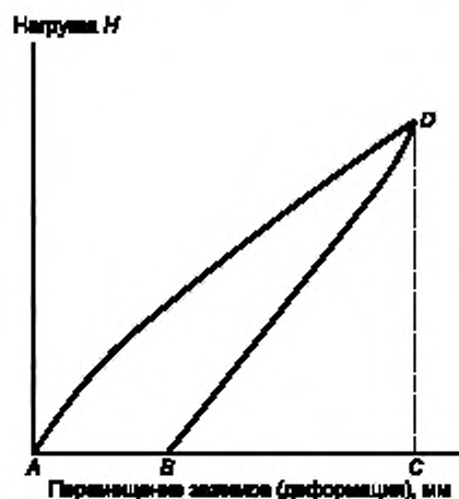
Рисунок А.1 — Кривая «нагрузка — деформация»
