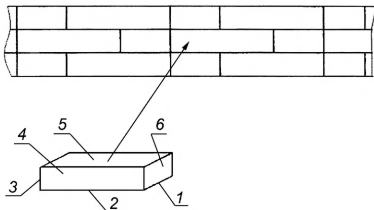
1 — ширина (толщина); 2 — длина; 3 — высота; 4 — ложок; 5 — постель; 6 — тычок
