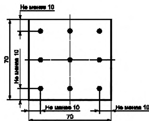
Рисунок 1 — Точки измерения толщины образца
