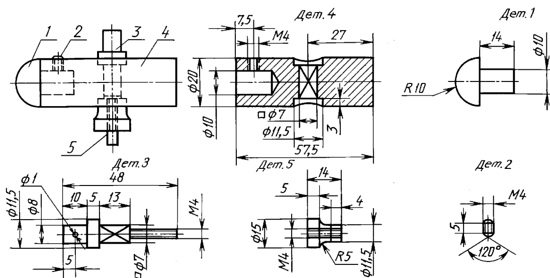
Материал деталей: 1 — полиамид; 2— 5 — сталь
