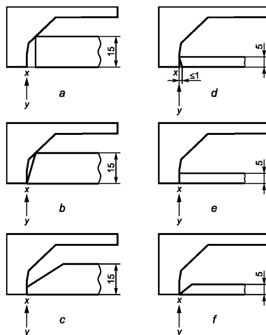
Случаи а) и б) — не соответствуют; случаи с), d), e) и f) — соответствуют (соответствие должно быть проверено требованиями 20.8, используя калибр, представленный на рисунке 23)
