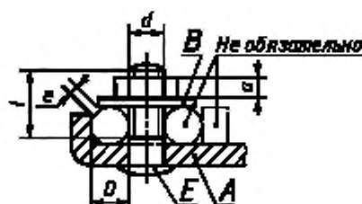
Болтовые выводы
