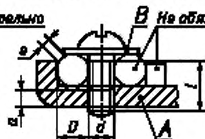
Винтовые выводы
