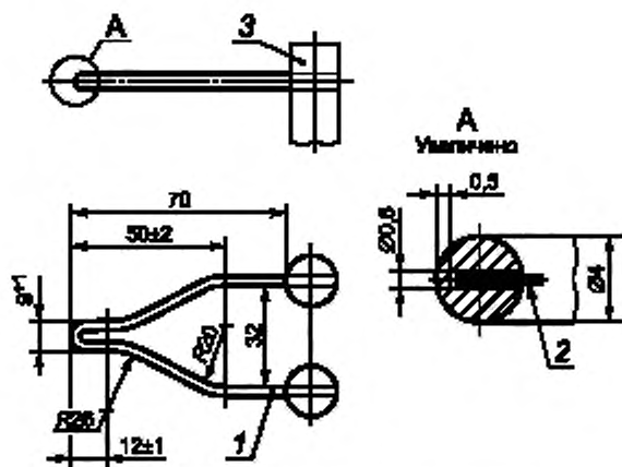
1 — расклеванная петля, запаянная в стойки; 2 — термопара; 3 — стойка
