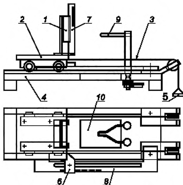
1 — фиксатор образца; 2 — каретка; 3 — шнур натяжения; 4 — основание; 5 — груз; 6 — скоб; 7 — шкала измерения пламени; 8 — шкала измерения глубины проникновения; 9 — раскаленная петля; 10 — отверстие в основании для падения продуктов горения
