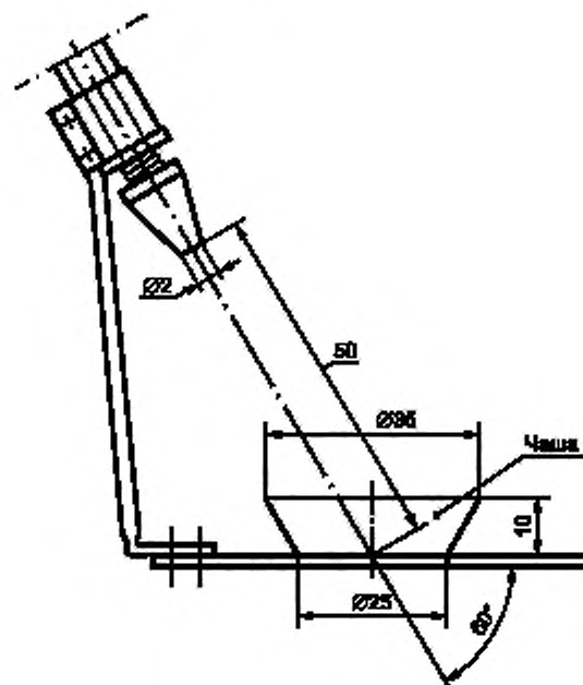
Рисунок 4 — Разбрызгиватель
