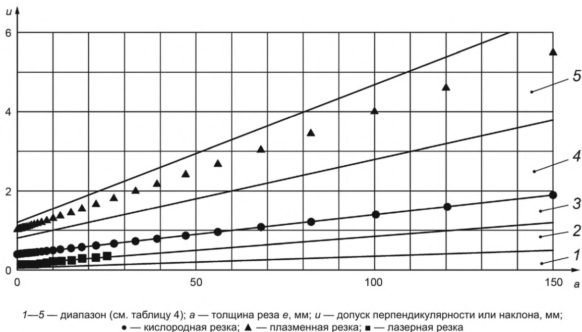
Рисунок А.2 — Стандартное качество реза, получаемое при допуске перпендикулярности или наклона u (толщина вырезаемой детали до 150 мм)
