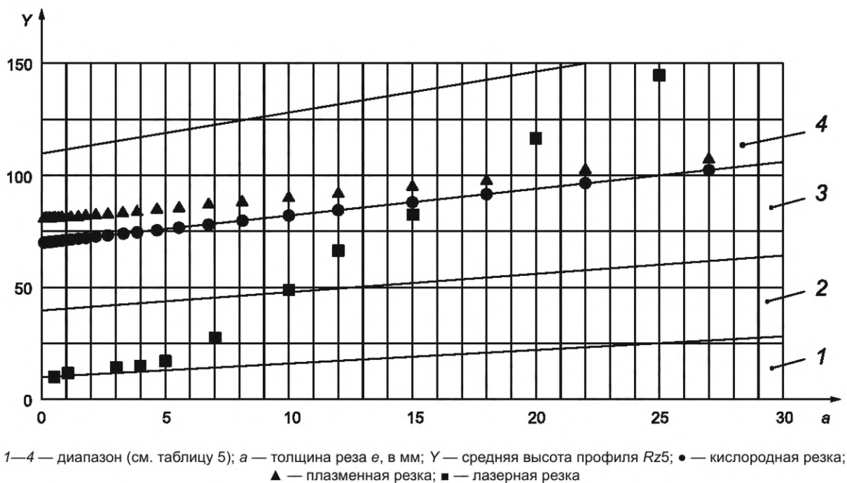
Рисунок А.3 — Стандартное качество реза, получаемое при средней высоте профиля Rz5 (толщина вырезаемой детали до 30 мм)
