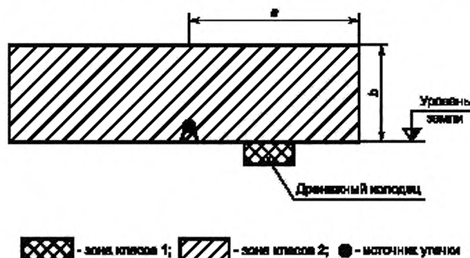
Пример № 1 Насос для перекачки горючей жидкости, установленный снаружи на уровне земли
