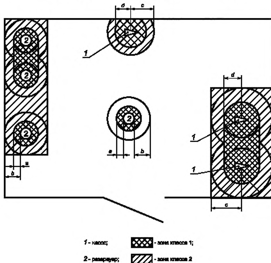
Пример № 10 Помещение для смешивания красок в цеху по производству красок
