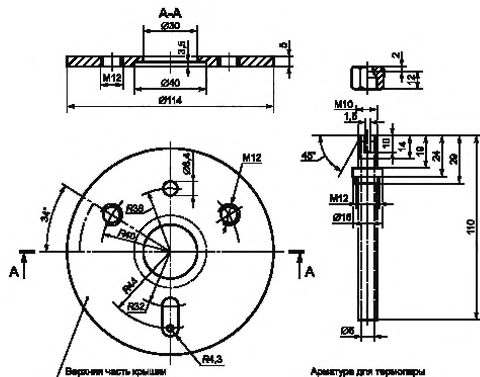
Рисунок А.8 — Крыка стального цилиндра
