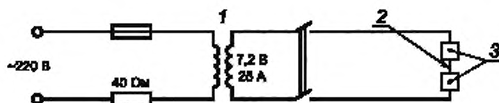
1 — трансформатор с площадью поперечного сечения сердечника 19 см 2 ; 2 — вольфрамовая проволока; 3 — медные бруски
