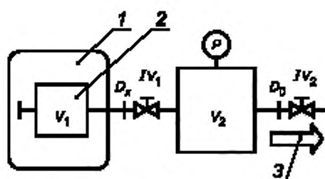
1 — система, заполненная гелием; 2 — испытываемая система; 3 — выход
