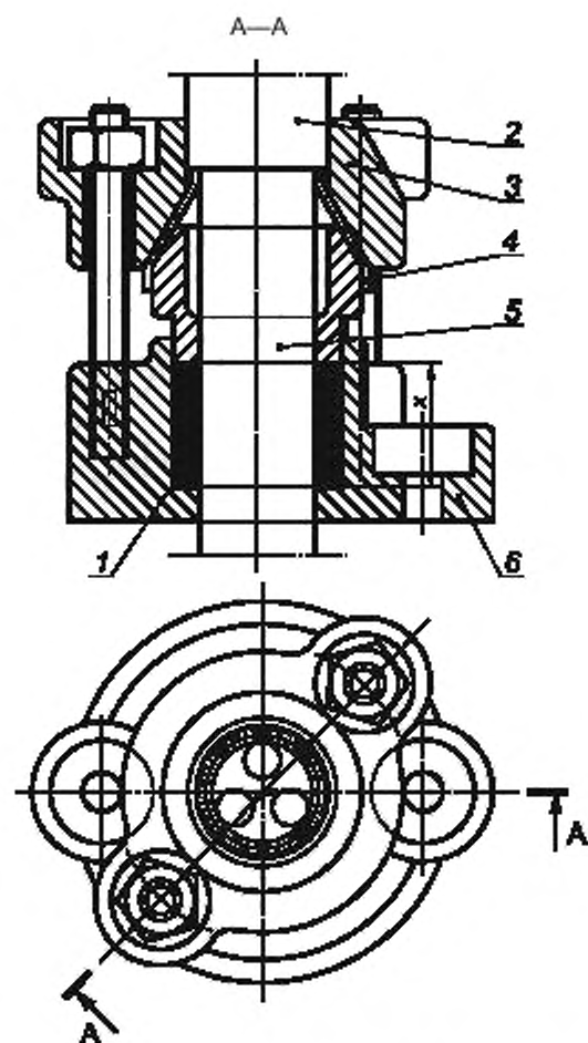
1 — уплотнительное кольцо; 2 — внешняя оболочка кабеля; 3 — зажим для крепления брони; 4 — броня; 5 — внутренняя оболочка кабеля; 6 — фланец для крепления к корпусу оболочки, x — осевая высота уплотнительного кольца измеряется после сжатия
