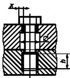
\sigma — отверстие со стандартным зазором для прохода резьбы соответствующей формы. Размер h должен быть не более основного диаметра резьбы крепежной детали. X — опорный размер крепежной детали с уменьшенным телом, он должен быть не более значения опорного размера стандартной головки стандартной крепежной детали (с полным телом) с резьбой используемого размера по всей длине.
