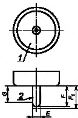
Рисунок И.1 – Одноштырьковый патрон типа Fa6
