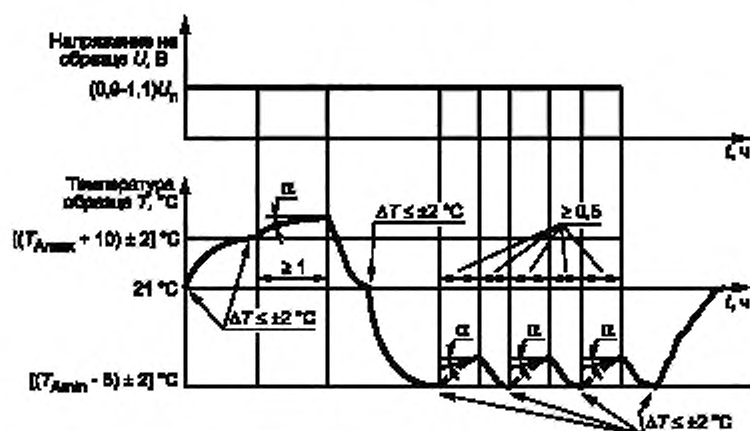
Схема теплового циклического испытания согласно 8.2.1.2
