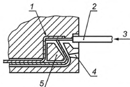
1 — токоведущий проводник; 2 — участок проводника для испытания растягивающим усилием; 3 — проводник, рассчитанный на максимальный ток 3А; 4 — устройство разъединения; 5 — ограничитель
