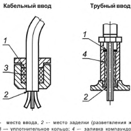
Рисунок 2 — Место ввода и заделки кабеля (разветвления жил)
