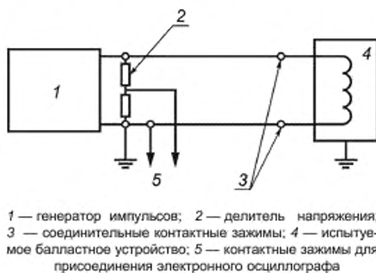
Рисунок 5 — Электрическая схема установки для испытаний импульсом высокого напряжения
