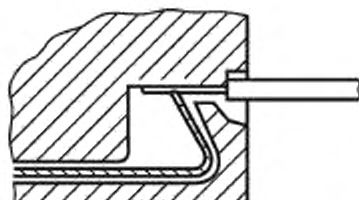
Рисунок 4б — Пример недопустимого для использования невинтового пружинного лепесткового зажима
