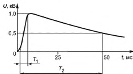
Рисунок 6 — Импульс высокого напряжения
