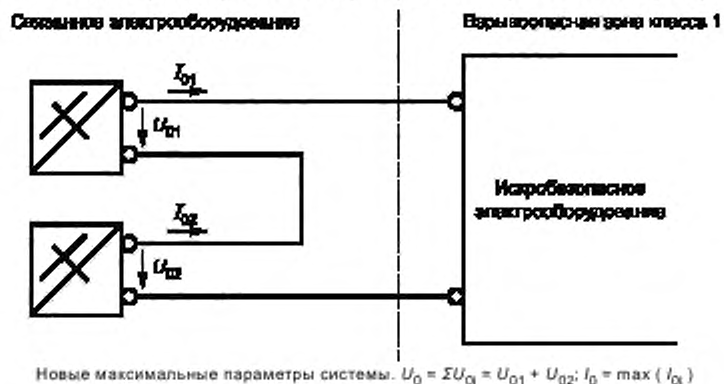
Рисунок В.1 – Последовательное соединение. Суммирование напряжений
