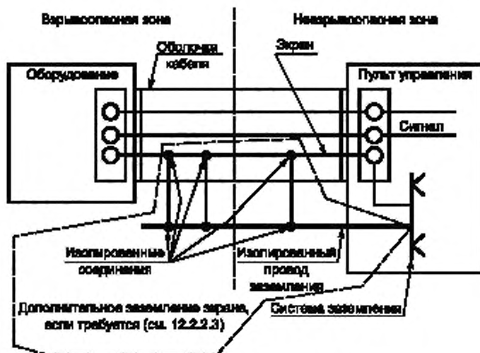
Рисунок 2 - Заземление проводящих экранов
