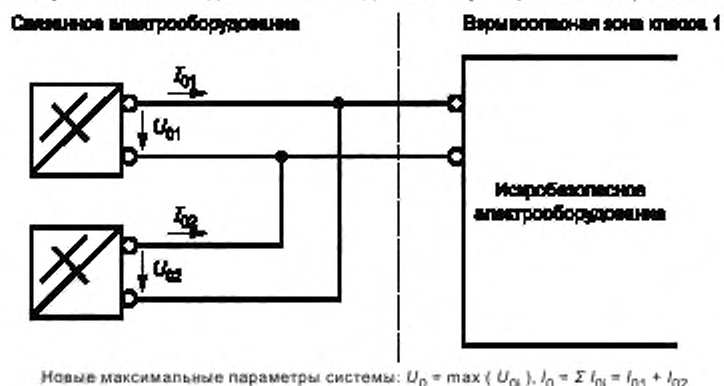
Рисунок В.2 – Параллельное соединение. Суммирование токов
