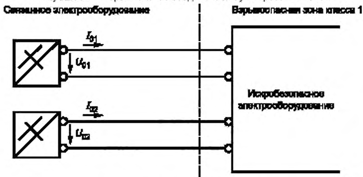
Рисунок В.2 – Параллельное соединение. Суммирование токов
