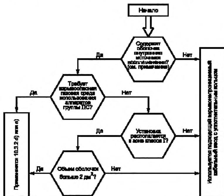
Рисунок 1 – Схема выбора кабельного ввода во взрывонепроницаемые оболочки для кабелей в соответствии с 10.3.2 б).
