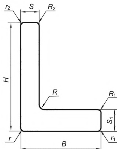
Рисунок 1 — Прессованный прямоугольный профиль неравнополочного углового сечения
