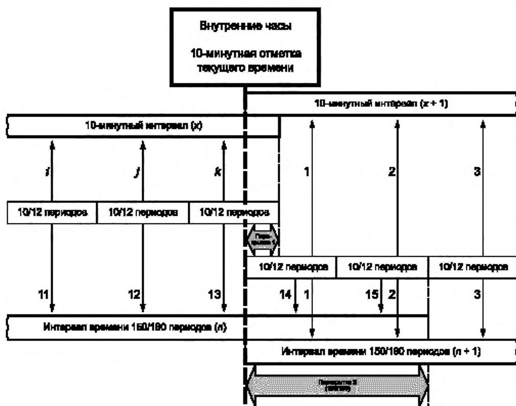
Рисунок 2 — Синхронизация объединенных интервалов для класса А
