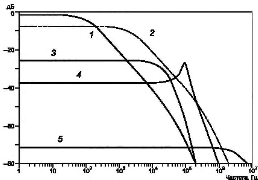
1 — испытательный сигнал 10 мкс (длительность фронта)/1000 мкс (длительность импульса); 2 — микросекундная импульсная помеха большой энергии (импульс напряжения 1/50 мкс); 3 — микросекундная импульсная помеха большой энергии (импульс тока 6,4/16 мкс); 4 — одиночная колебательная затухающая помеха с частотой колебаний 100 кГц; 5 — пакеты наносекундных импульсных помех 5/50 нс
