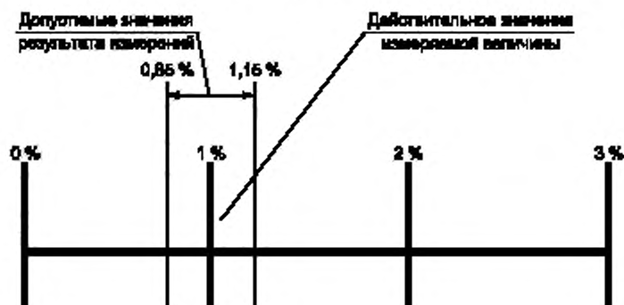
Рисунок 5 — Пример неопределенности измерений несимметрии напряжений
