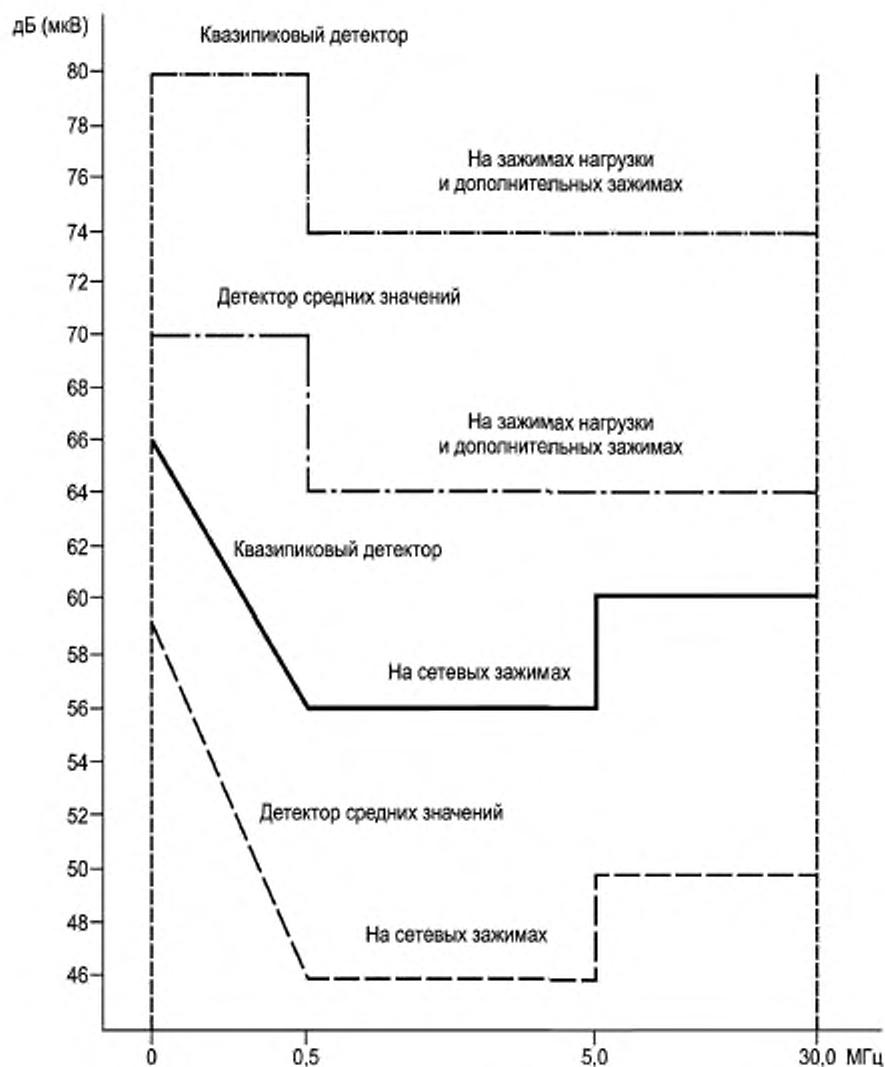
Рисунок 2 — Значения норм напряжения ИРП на зажимах ТС в полосе частот от 148,5 кГц до 30 МГц для регулирующих устройств
