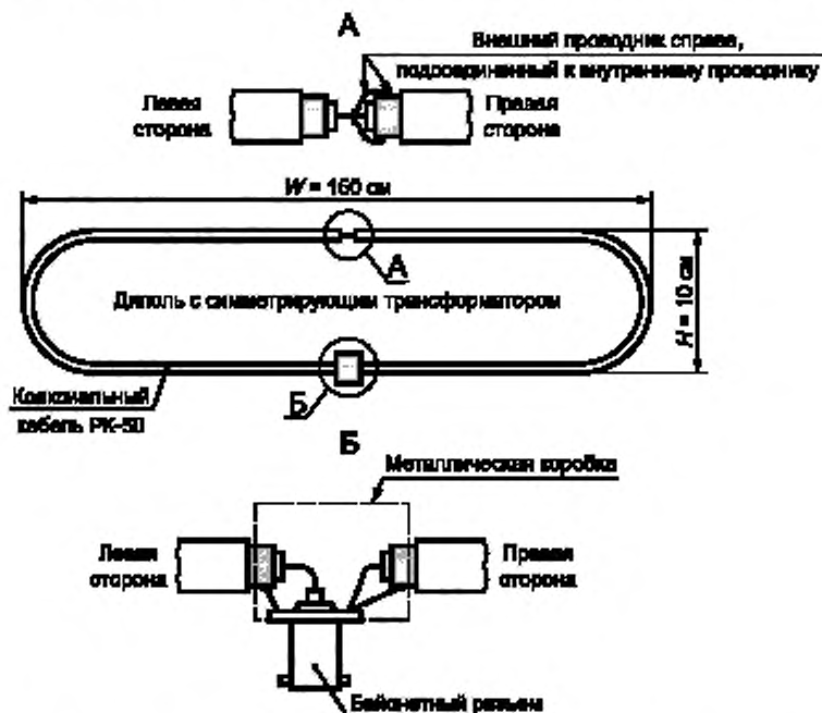
Рисунок В.9 — Конструкция диполя с симметрирующим трансформатором
