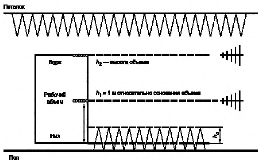
Рисунок 16 — Позиции при измерении КСВ Н в горизонтальной плоскости (см. 8.2.2.2.1)
