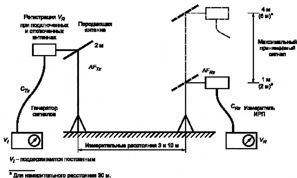
Рисунок 4 — Расположение оборудования для измерения затухания площадки при горизонтальной поляризации (см. 5.6 и приложение E)
