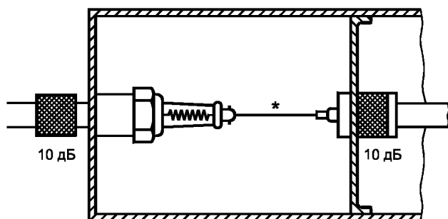
Рисунок В.7 — Помехоподавляющая свеча зажигания
