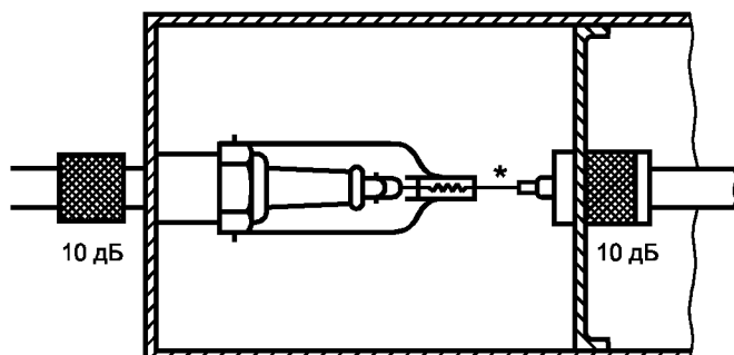
Рисунок В.5 — Прямое помехоподавляющее устройство системы зажигания со свечей зажигания (экранированное или неэкранированное)
