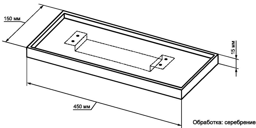
Рисунок В.3 — Детали крышки испытательного контейнера
