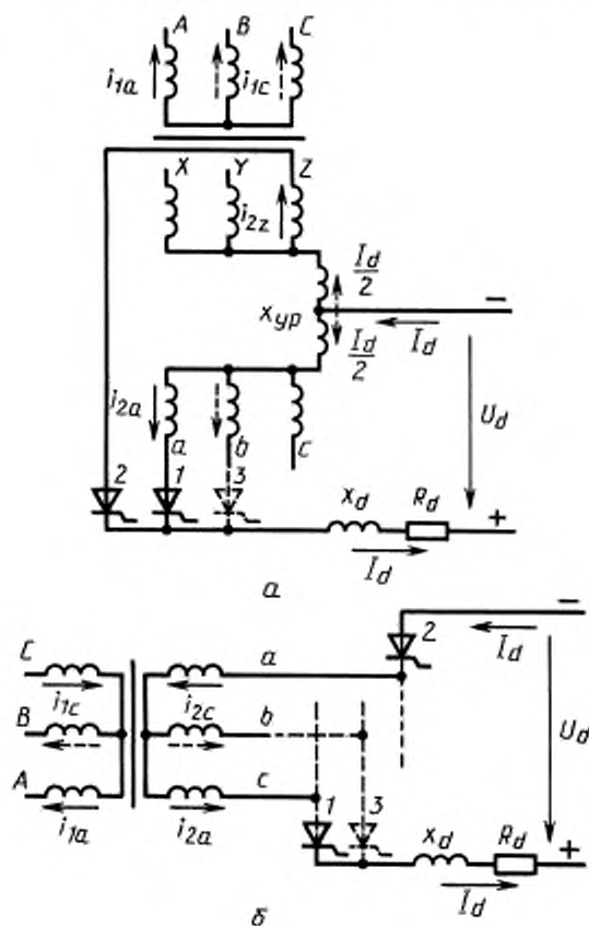
а — две обратные звезды с уравнительным реактором; б — трехфазная мостовая
