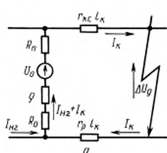
Схемы замещения цепи КЗ при повреждении в контактной сети тяговых (железнодорожных) подстанций
