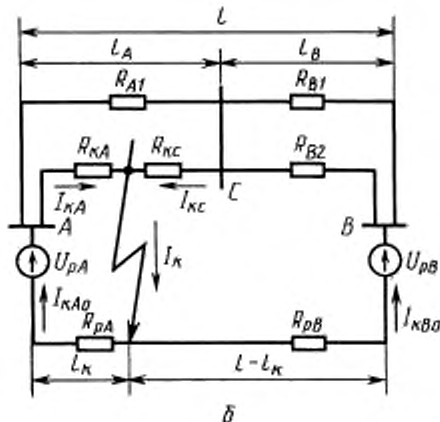
a — одностороннее питание контактной сети; б — двустороннее питание контактной сети на двухпутном участке с постом секционирования
