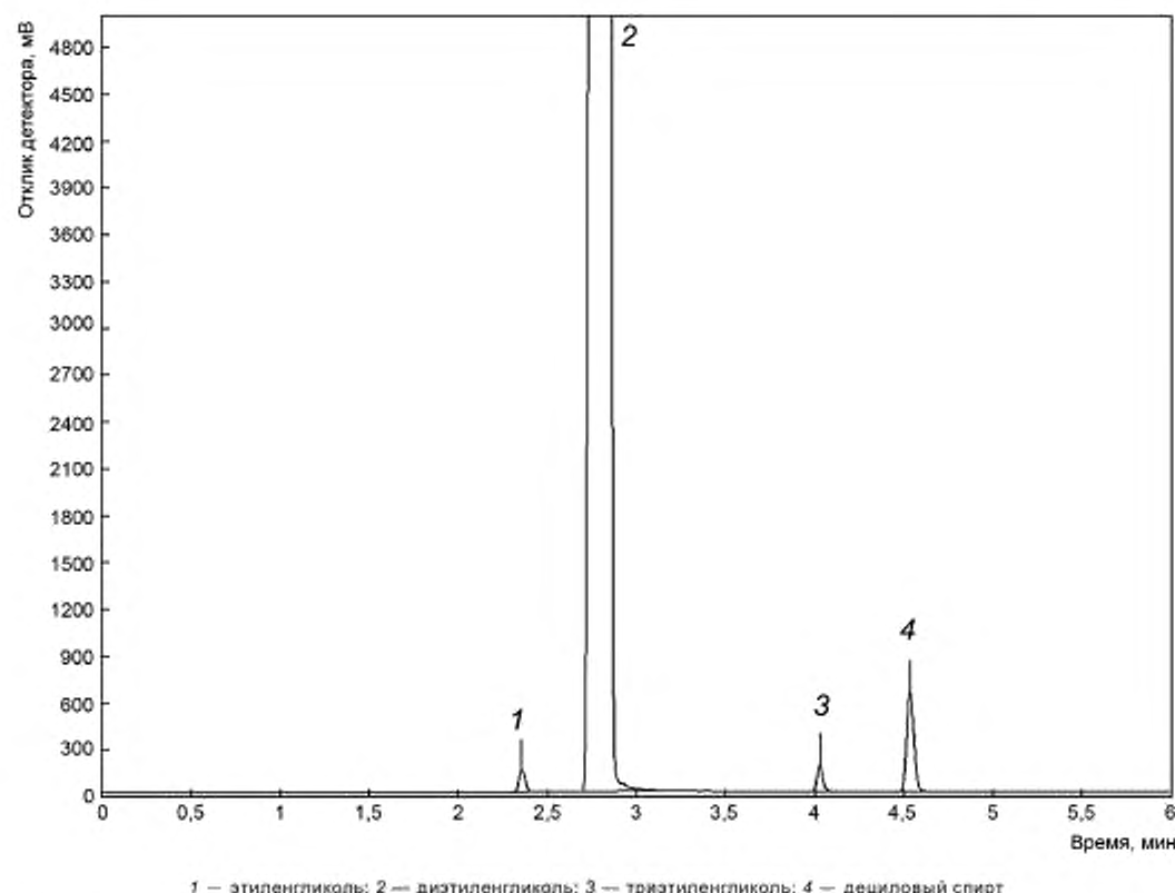
Рисунок 3 — Хроматограмма пробы товарного диэтиленгликоля на капиллярной колонке VERTICAL VertiBond-1
