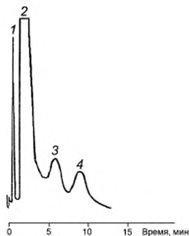
Рисунок 1 — Типовая хроматограмма органических примесей в диэтиленгликоле на колонке с насадкой I
