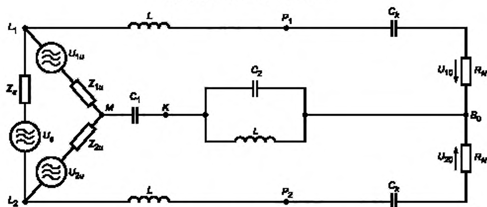
b) Эквивалентная схема источника ЭД-помех и схема измерения
