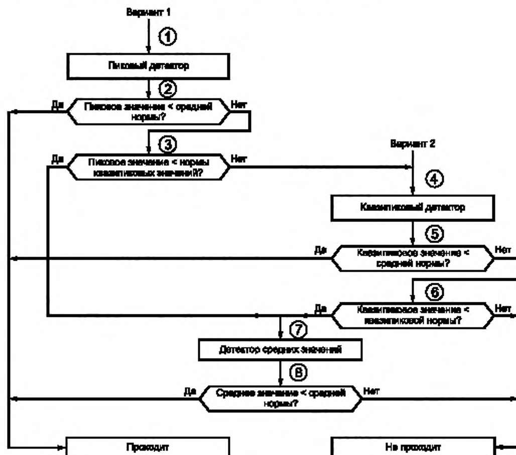
Рисунок С.1 — Алгоритмы определения соответствия ТС нормам кондуктивных ИРП при использовании пикового, квазипикового детектора и детектора средних значений
