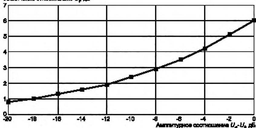
Рисунок А.10 — Увеличение пикового значения при суперпозиции двух немодулированных сигналов ( U_a — уровень посторонних радиопомех; U_i — уровень ИРП, создаваемых испытуемым ТС)
