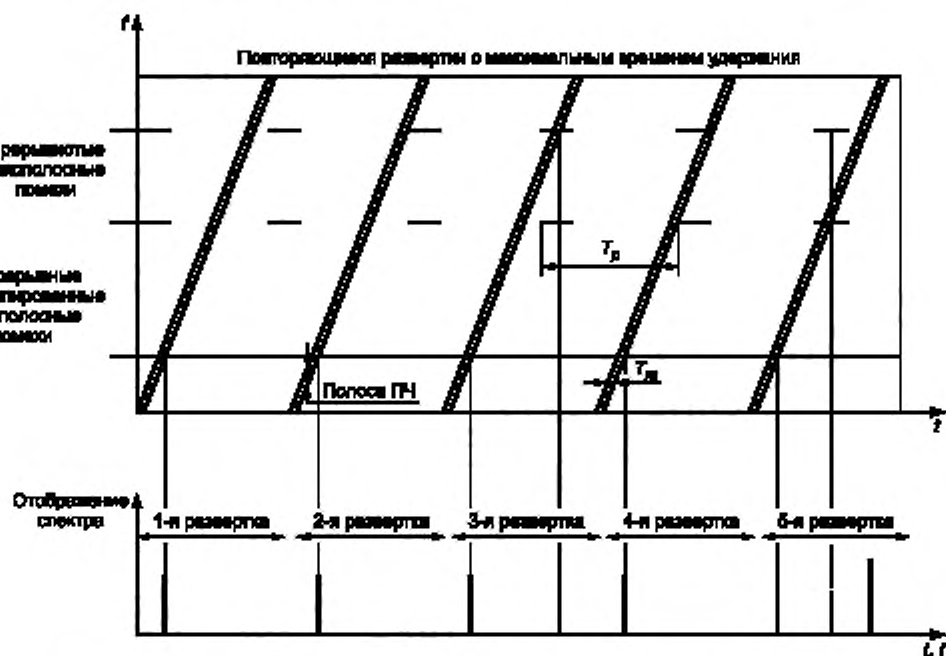
Рисунок 4 — Пример измерения прерывистых узкополосных ИРП с помощью быстрых коротких повторяющихся разверток и функций «фиксации максимума» для получения обзора спектра помехи
