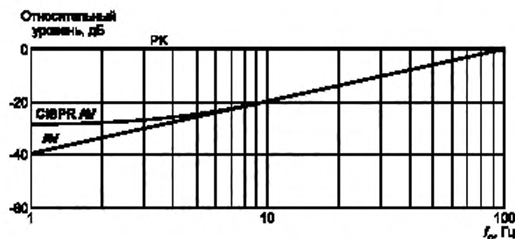
Рисунок D.2 — Весовая функция импульса 10 мс при детектировании пиковым детектором «РК», детектором средних значений при учете пиковых значений «CISPR AV» и детектором средних значений без учета пиковых значений «AV» для постоянной времени прибора 100 мс
