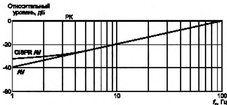
Рисунок D.1 — Весовая функция импульса 10 мс при детектировании пиковым детектором «РК», детектором средних значений при учете пиковых значений «CISPR AV» и детектором средних значений без учета пиковых значений «AV» для постоянной времени прибора 160 мс
