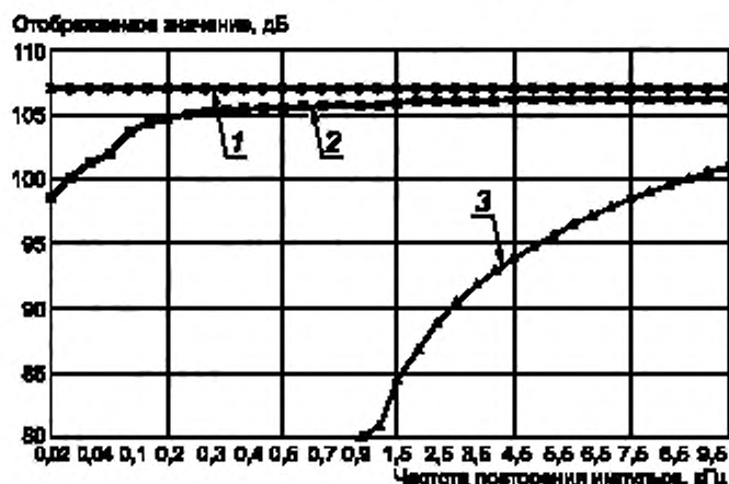
Рисунок А.6 — Напряжение импульсно-модулированного сигнала (ширина импульса 50 мкс) в функции от частоты повторения импульсов при использовании пикового, квазипикового детекторов и детектора средних значений
