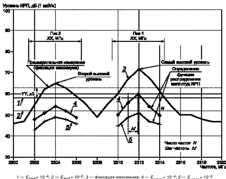
Рисунок Е.1 — Пример применения функции распределения амплитуд для флуктуирующих помех, метод 1
