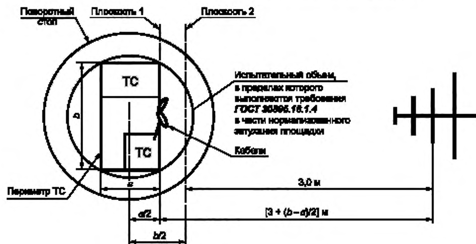
Рисунок 12 — Испытательная установка для напольных ТС, вид сверху
