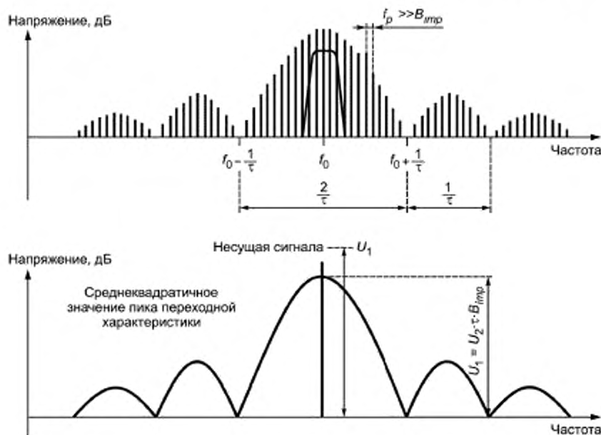
Рисунок Е.6 — Фильтрация, когда значение B_{\text{имп}} намного больше частоты повторения импульсов
