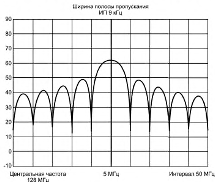
Рисунок Е.3 — Спектрограмма импульсно-модулированного сигнала при ширине импульсов 200 мс
