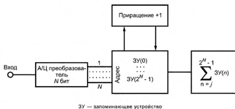
Рисунок G.2 — Блок-схема устройства измерения функции распределения амплитуд ИРП с аналого-цифровым преобразователем
