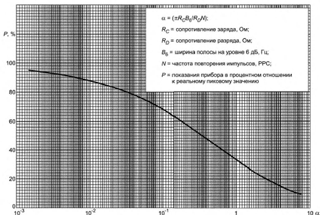
Рисунок E.2 — Коэффициент выпрямления импульсов P (показания прибора в процентном отношении к реальному пиковому значению)
