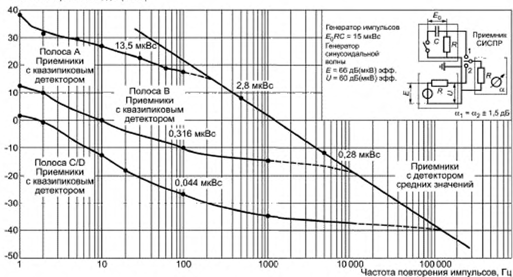
д) Теоретические кривые импульсной характеристики ИП с квазипиковым детектором и детектором средних значений (см. 6.4.2)
