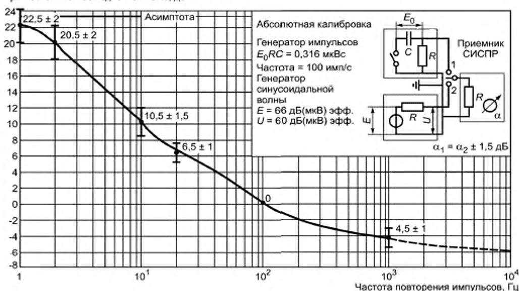
б) Импульсная характеристика ИП для полосы частот В (от 0,15 до 30 МГц) и допускаемые отклонения ее значений
