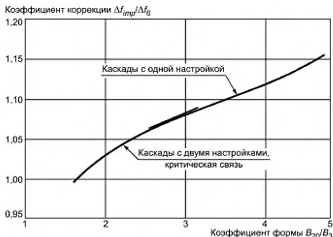
Рисунок Е.1 — Коэффициент коррекции для оценки отношения B_{imp}/B_8 для других типов настраиваемых схем
