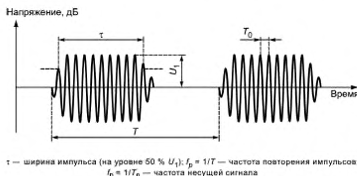
Рисунок Е.4 — Импульсно-модулированный ВЧ-сигнал, подаваемый на ИП
