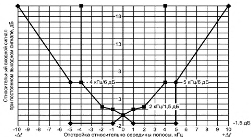
б) Пределы характеристики частотной избирательности ИП для полосы частот В (от 0,15 до 30 МГц)
