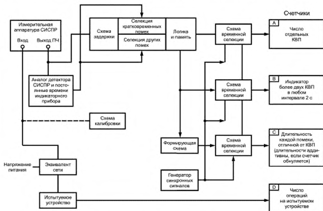
Рисунок 6 — Пример блок-схемы анализатора кратковременных ИРП
