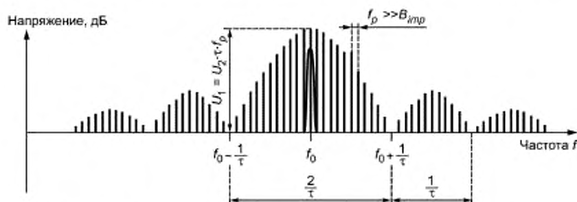
Рисунок Е.5 — Фильтрация, когда B_{\text{имп}} намного меньше частоты повторения импульсов
