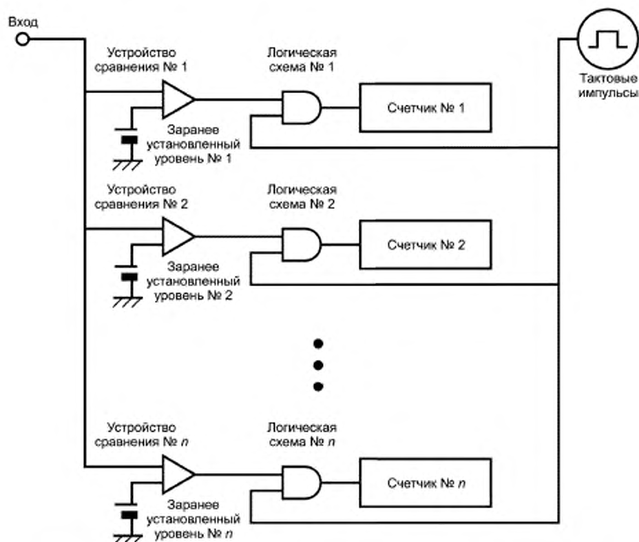
Рисунок G.1 — Блок-схема устройства измерения функции распределения амплитуд ИРП без аналого-цифрового преобразователя
