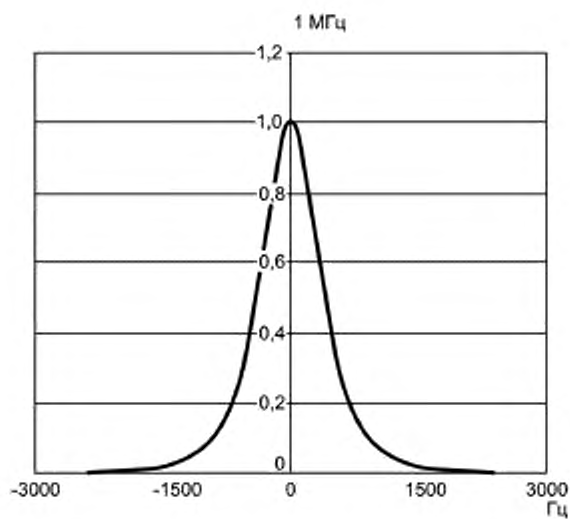
Рисунок Е.8 — Пример нормализованной линейной функции частотной избирательности
