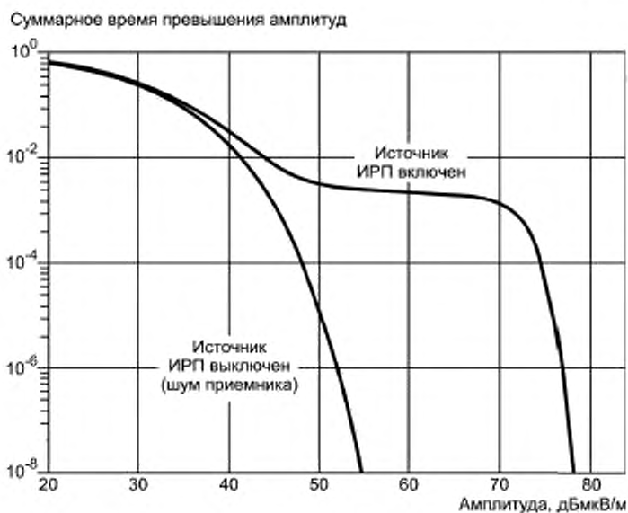
Рисунок G.3 — Пример функции распределения амплитуд ИРП
