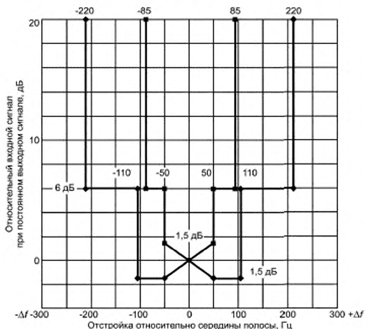
а) Пределы характеристики частотной избирательности ИП для полосы частот А (от 9 до 150 кГц)
