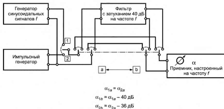
Рисунок 3 — Схема измерения ослабления продуктов интермодуляции
