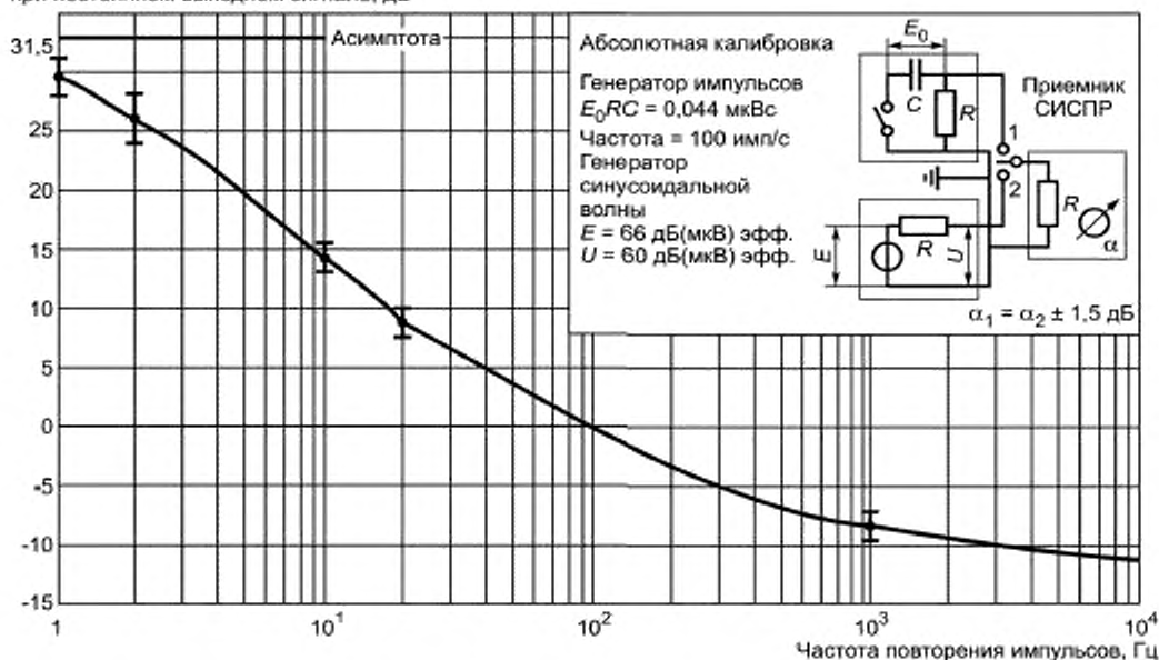
с) Импульсная характеристика ИП для полосы частот C/D (от 30 до 1000 МГц) и допускаемые отклонения ее значений
