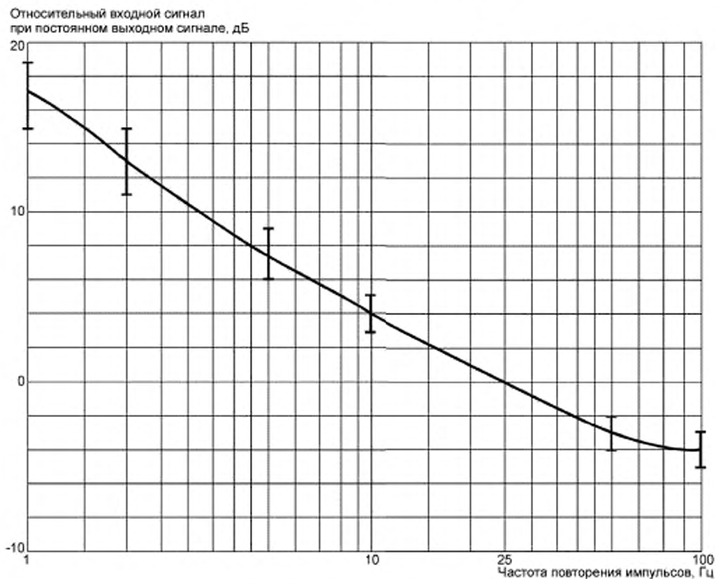
а) Импульсная характеристика ИП для полосы частот А (от 9 до 150 кГц) и допускаемые отклонения ее значений
