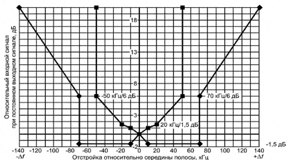
с) Пределы характеристики частотной избирательности ИП для полос частот С и D (от 30 до 1000 МГц)
