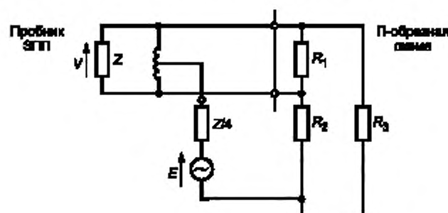
Рисунок Е.2 — Схема измерения входного полного сопротивления
