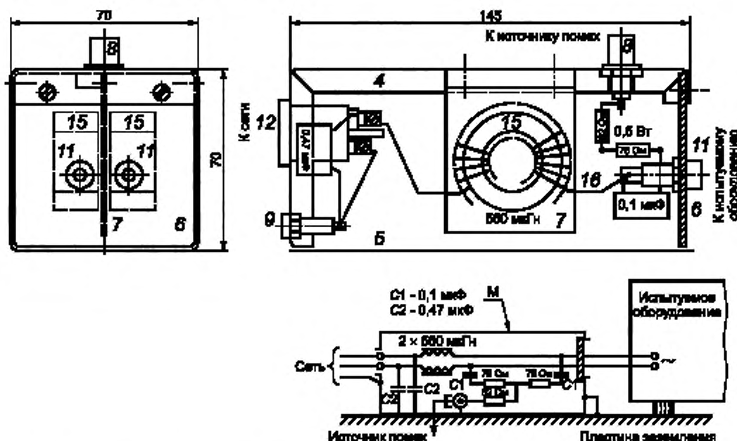
4—9 — см. блок связи типа А; 11 — сетевое гнездо для испытываемого оборудования (два изолированных однополюсных гнезда); 12 — сетевая штепсельная вилка (2Р + земля); 15 — два дросселя из склеенных ферритовых колец типа 4С6, \varphi = 36 мм, внутренний диаметр 23 мм, толщина 30 мм с 40 витками на каждом; 16 — изолированный медный провод с внешним диаметром 1,5 мм
