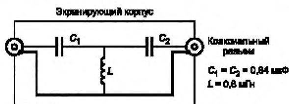
Рисунок В.2 — Схема фильтра высоких частот с частотой среза 9 кГц
