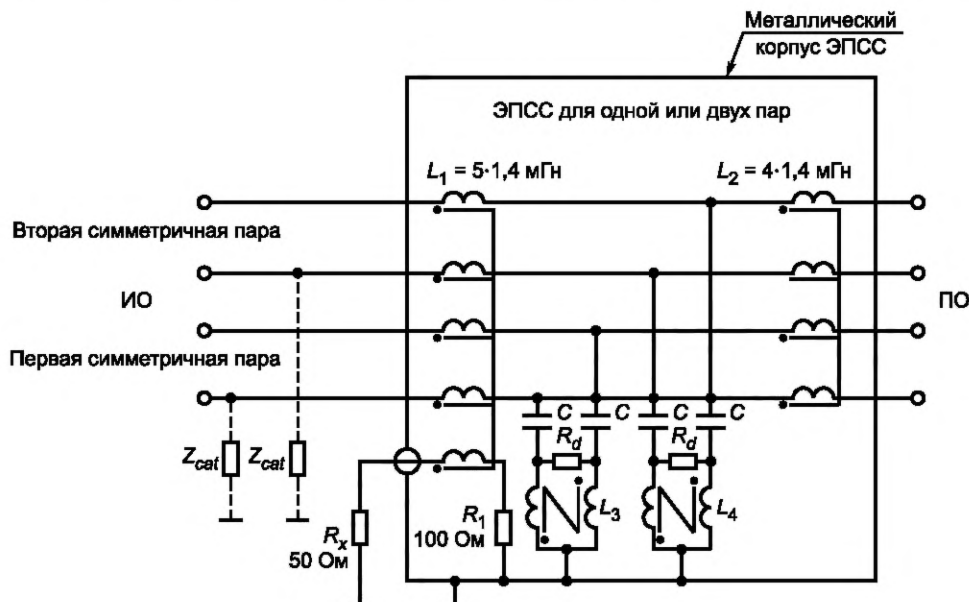
Рисунок D.1 — ЭПСС для применения с одной незэкранированной симметричной парой
