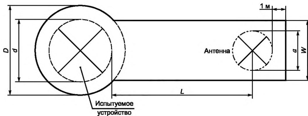
Рисунок 3 — Минимальный размер металлической пластины заземления
