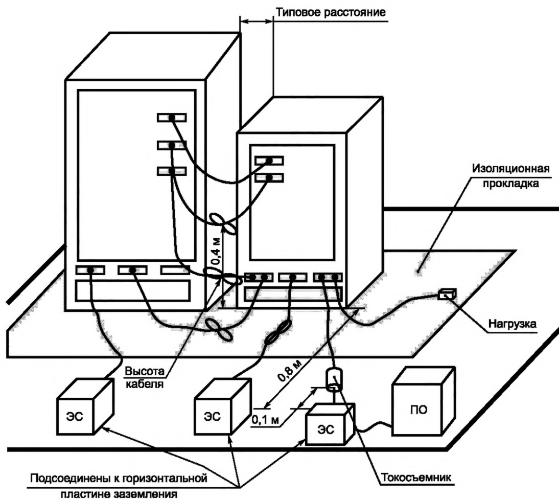
Рисунок 8 — Размещение ИО: напольное оборудование, измерение кондуктивных ИРП
