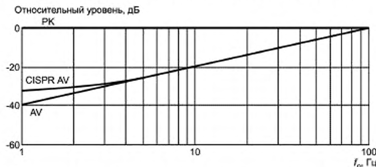
Рисунок С.1 — Веса функции импульса 10 мс при детектировании пиковым детектором «PK», детектором средних значений при учете пиковых значений «CISPR AV» и детектором средних значений без учета пиковых значений «AV» для постоянной времени прибора 160 мс
