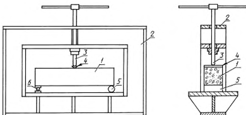
1 — образец; 2 — нагружающее устройство; 3 — нагружающий винтовой силоизмерительный шток; 4 — распределительная балка; 5 — роликовая опора; 6 — шарнирная опора
