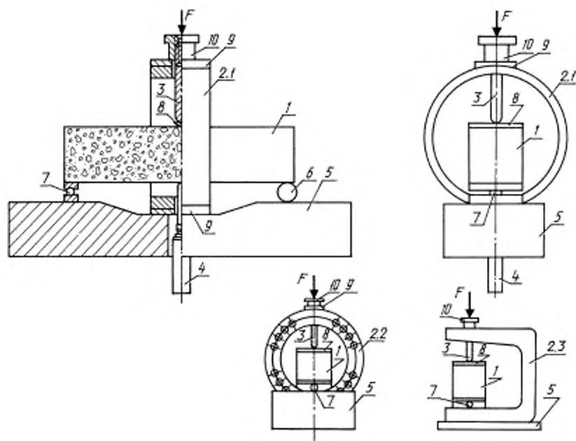
1 — образец; 2 — дополнительное перераспределяющее устройство типа: «кольцо» (2.1), «кольцо в кольцо» (2.2), «скоба» (2.3); 3 — нагружающий силоизмерительный шток; 4 — датчик перемещений; 5 — станина; 6 — роликовая опора; 7 — шарнирная опора; 8 — распределительная балка; 9 — фиксирующие накладки; 10 — фиксатор нагружающего силоизмерительного штока
