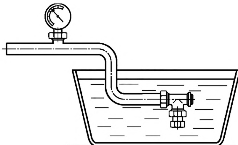
Рисунок 11 — Испытание герметичности уплотнения штока клапана
