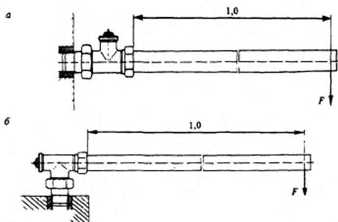
a — проходной клапан; б — угловой клапан
