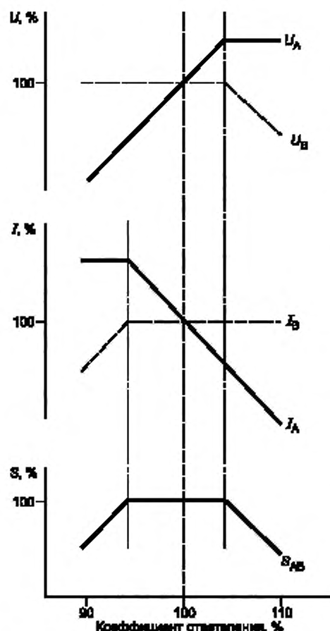
Рисунок 3 — Комбинированное регулирование напряжения (режим а)
