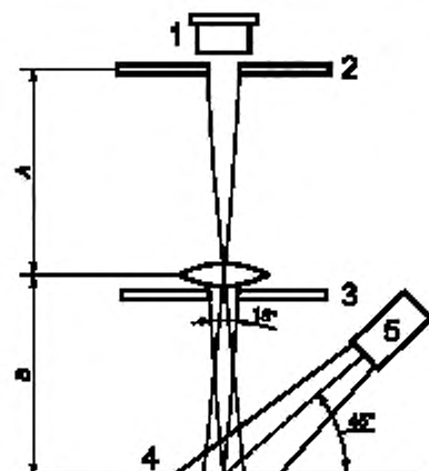
1 — фотоувеличивающий элемент; 2 — апертура при линейном увеличении 1:1 (размер A равен размеру B ); 3 — диафрагма; 4 — образец; 5 — источник оптического излучения
