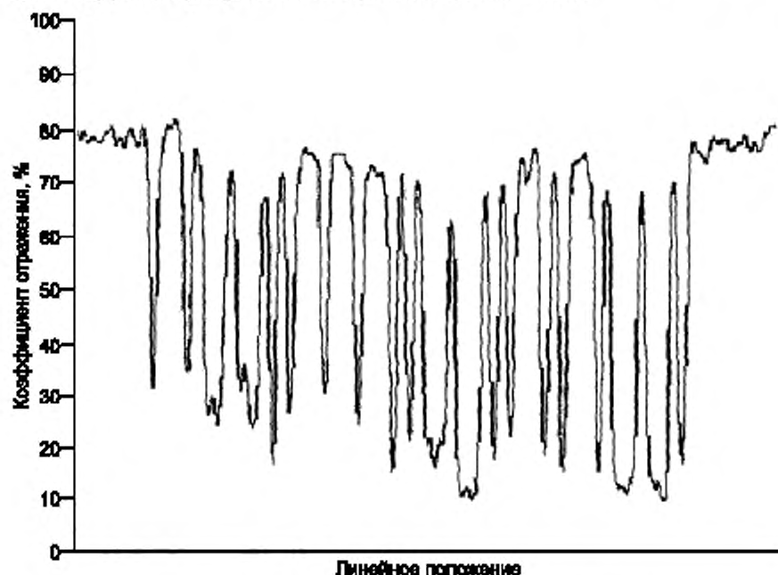
Рисунок 3 — Профиль отражения при сканировании
