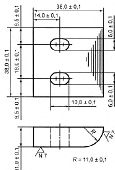
Рисунок 2 — Стальной нож
