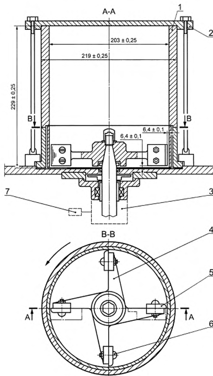
Рисунок 1 — Лабораторная мельница
