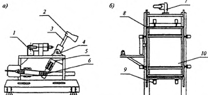
1 — высвобождающий механизм; 2 — головка топора; 3 — рукоятка; 4 — ось вращения; 5 — зажимное приспособление; 6 — натяжная пружина; 7 — регулятор высоты; 8 — зажимная рама; 9 — пневматические зажимы; 10 — испытываемый образец
