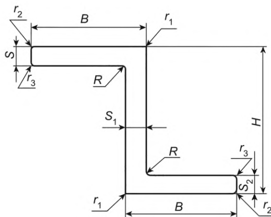
Рисунок 1 — Прессованный прямоугольный профиль равнополочного зетового сечения
