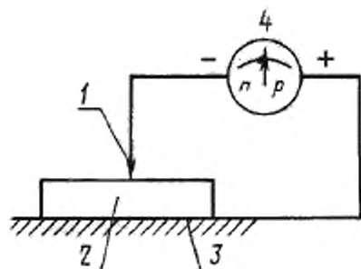
1 — зонд; 2 — образец; 3 — металлическая пластина; 4 — нуль-индикатор
