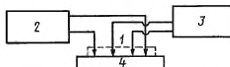
Блок-схема установки для измерения удельного электрического сопротивления
