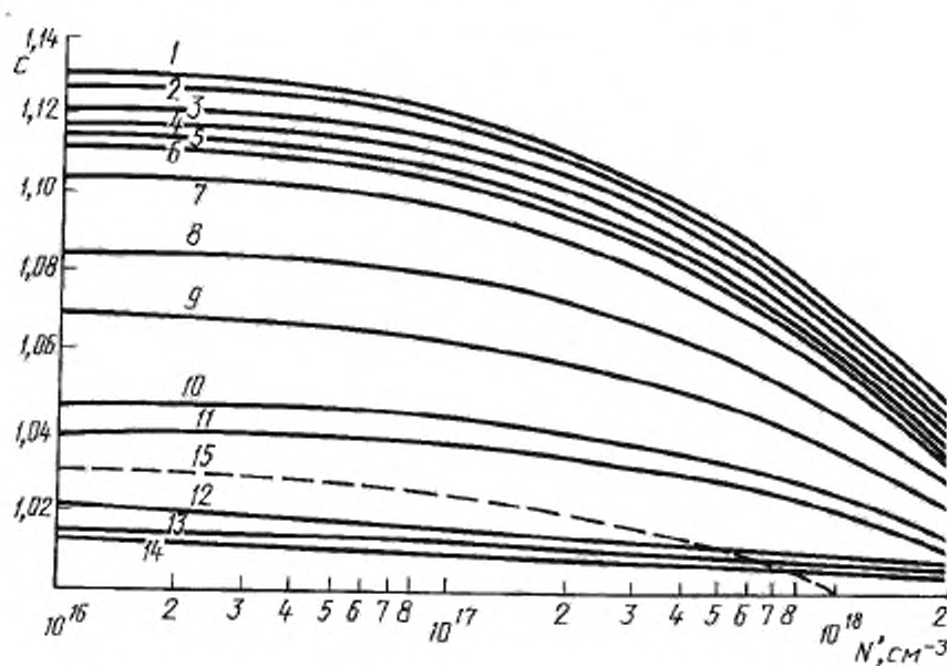
Зависимость коэффициента C от N' различных значений УЭС образцов ( n -Si) при проведении измерений дифференциальным методом
