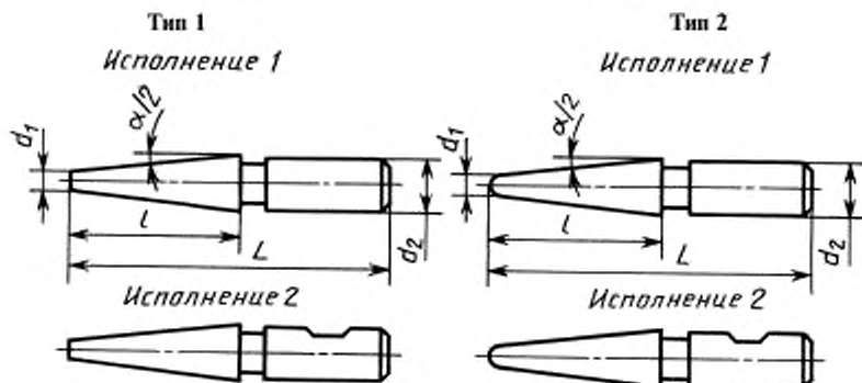
Размеры, мм
