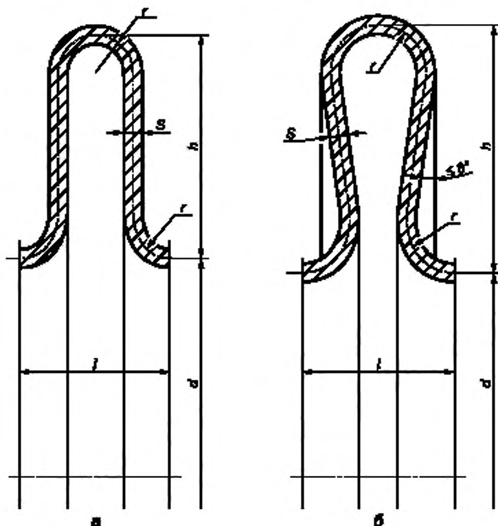
Рисунок 1 — Модели компенсаторов
