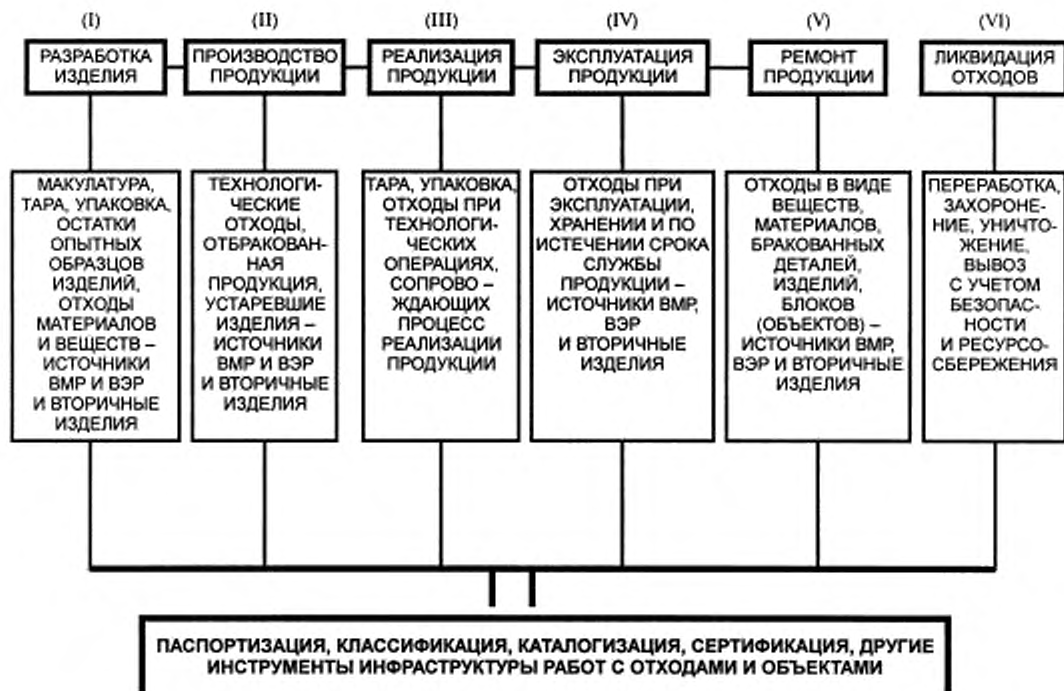
Схема образования и ликвидации основных видов объектов и отходов на стадиях жизненного цикла продукции (изделия)
