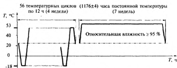
Рисунок А.1 — График испытаний стеклопакетов по режиму IV
